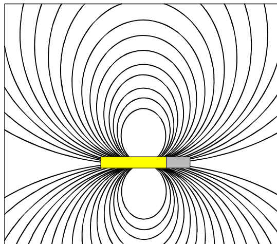
Forme elliptique du champ de signal de l'émetteur
