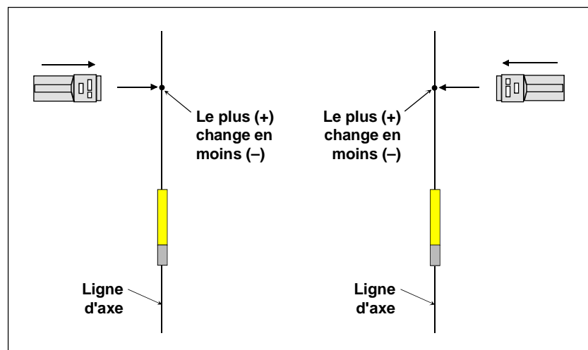
Test d'équilibre du récepteur – Vérifier que « + » devient « - » sur la même ligne en venant des deux directions.
