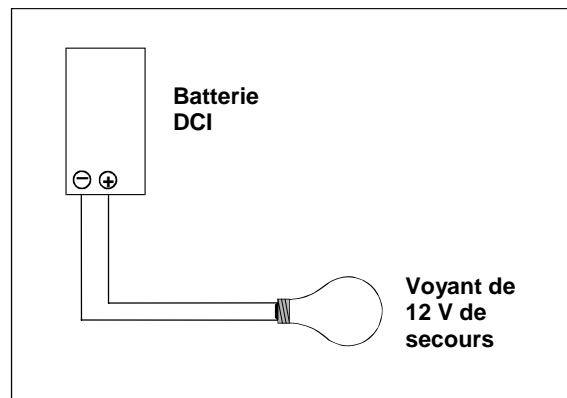
Branchement pour décharger manuellement une batterie
