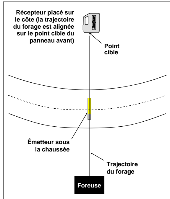
Mise en place du récepteur DigiTrak pour téleguidage
