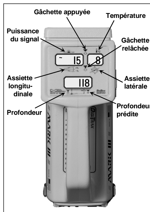
Récepteur DigiTrak – Vue des icônes des écrans d'affichage supérieurs
