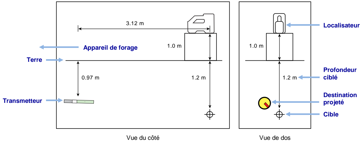
Transmetteur, Cible et Localisateur Élevé
