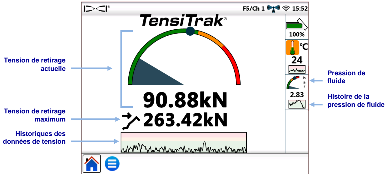
Gauge de TensiTrak
