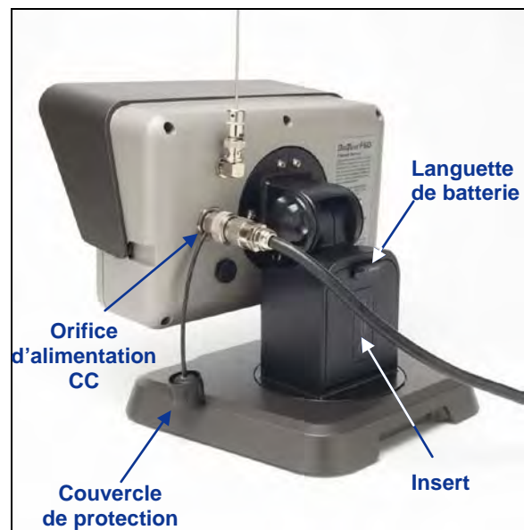
Câble d'alimentation CC et insert installés sur la visualisation à distance FSD
