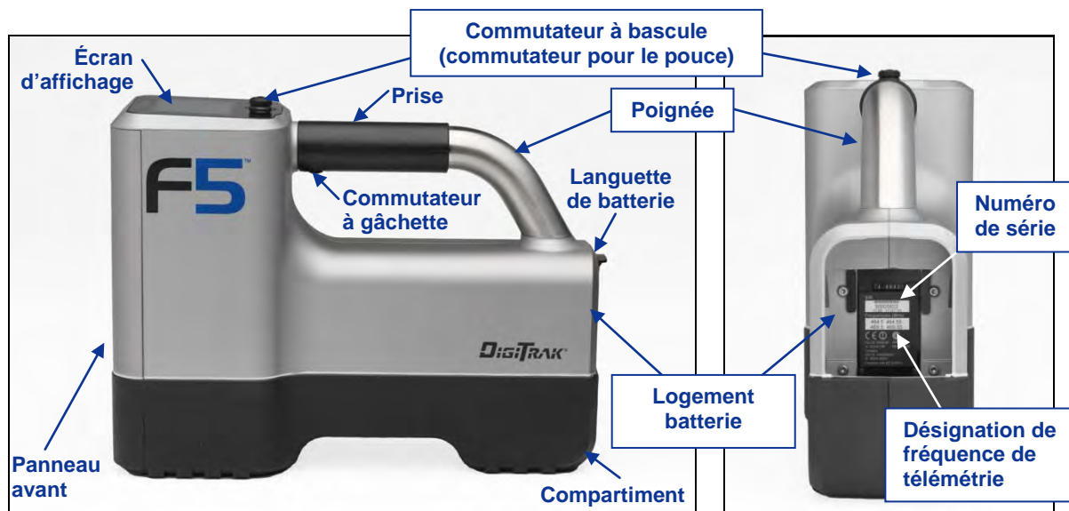
Récepteur F5 – Vues latérale et arrière
