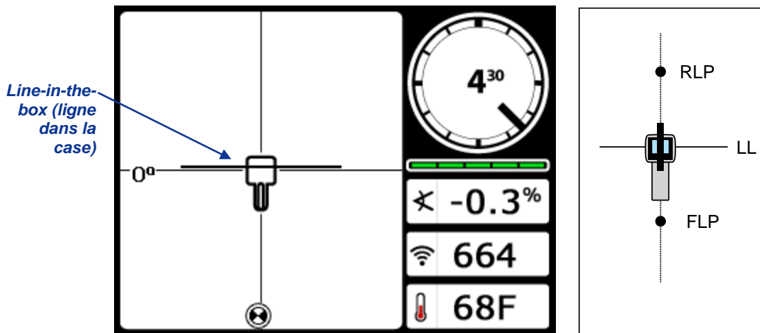
Écran mode localisation du récepteur (à l'axe LL)
