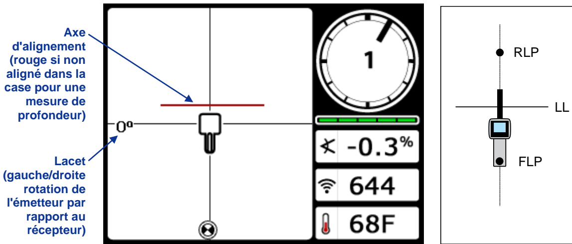
Écran mode localisation du récepteur (en se rapprochant de l'axe LL)
